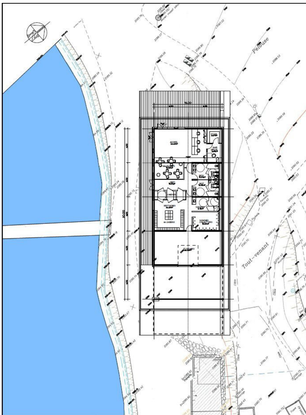
Figure 1. Copie du plan masse établi par l'architecte.
